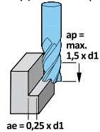
Konturenfräsen (3/4-Schneiden)
