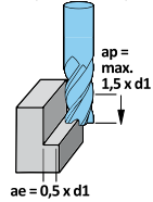
Konturenfräsen (2-Schneiden)
